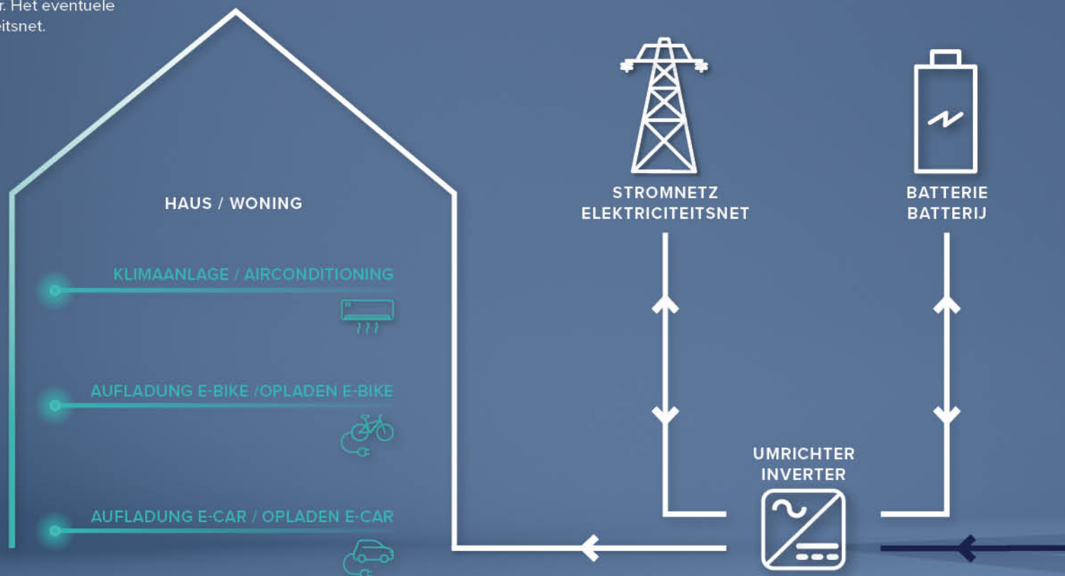
Elektrische Anlage Wohnhaus* / elektrische installatie woning*
